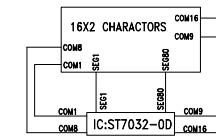
COM &amp; SEG LAYOUT
