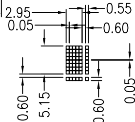
DOT DETAIL:
