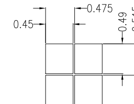
DOTS SIZE SCALE: 20:1
