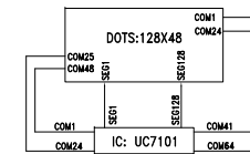
COM & SEG LAYOUT
