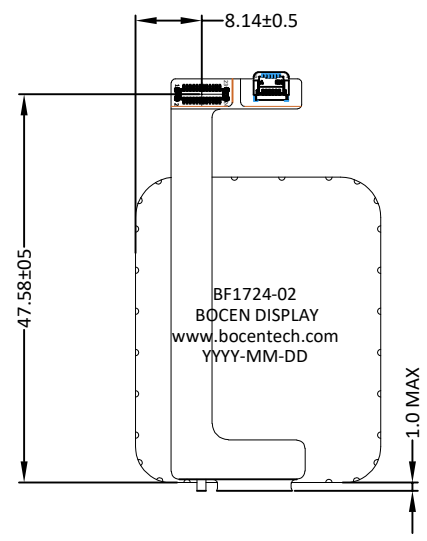
FPC弯折示意图 FPC展开出货
