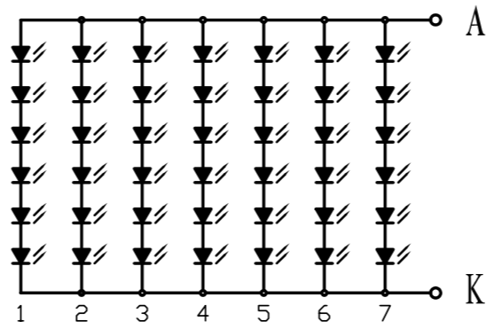
LED 电路图
