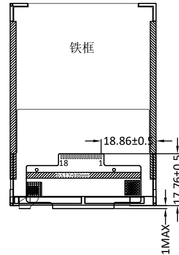
FPC弯折示意图 FPC展开出货
