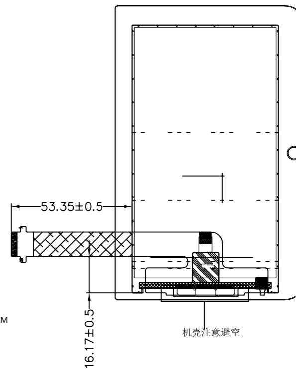
FPC弯折示意图 弯折出货
