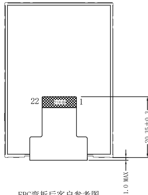
FPC弯折后客户参考图 展开出货
